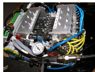
Bloc commande de harpe automatique
